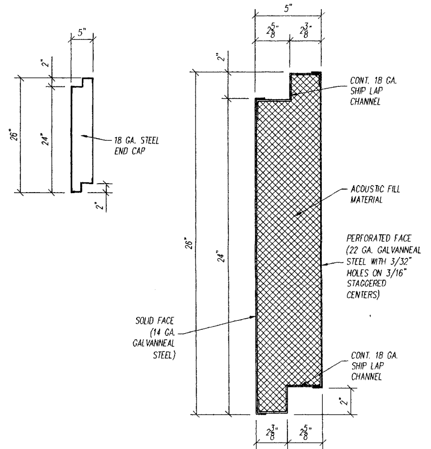
SECTION A-A
